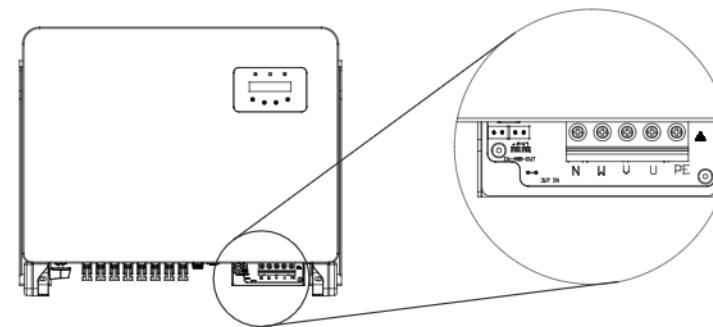
Figura 5.19 fiação
