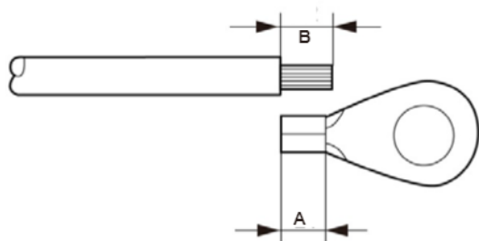
Figura 5.7 Comprimento adequado
