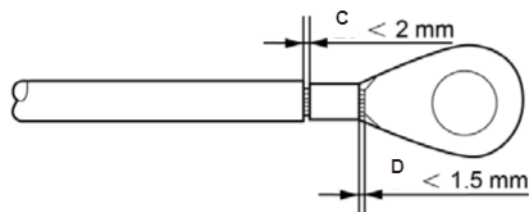
Figura 5.8 Fio descarnado
