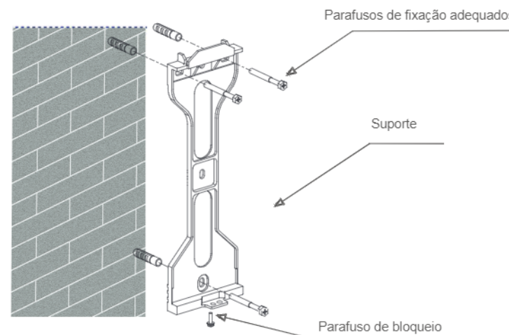
▲ Figura 4.4 Montagem do inversor na parede
