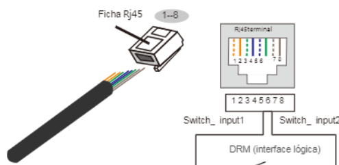
▲ Figura 4.29 Retire a camada de isolamento e ligue à ficha RJ45 3. Ligue o
