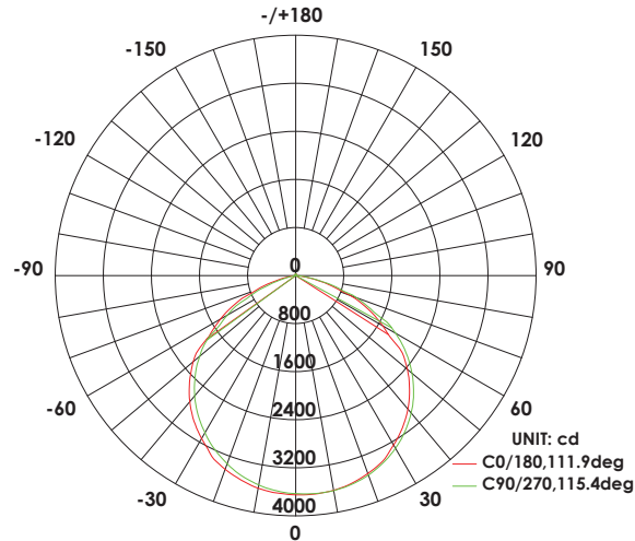
Curva Fotométrica
